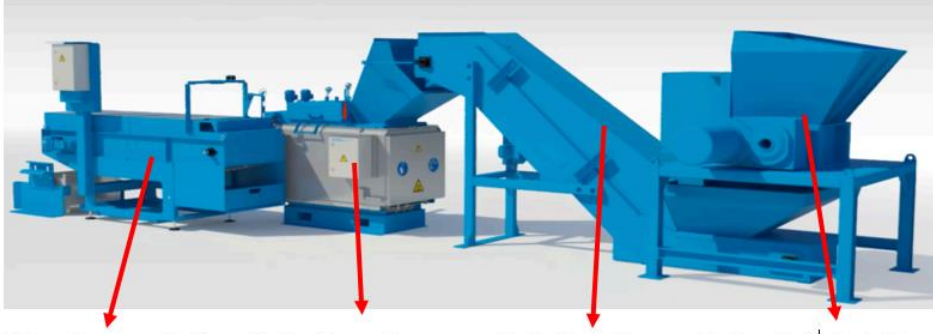
5. K l e Konvey r  4. Ergitme Fırını 3. Yolluk Konvey r  2. Yolluk Kırma Mak.
