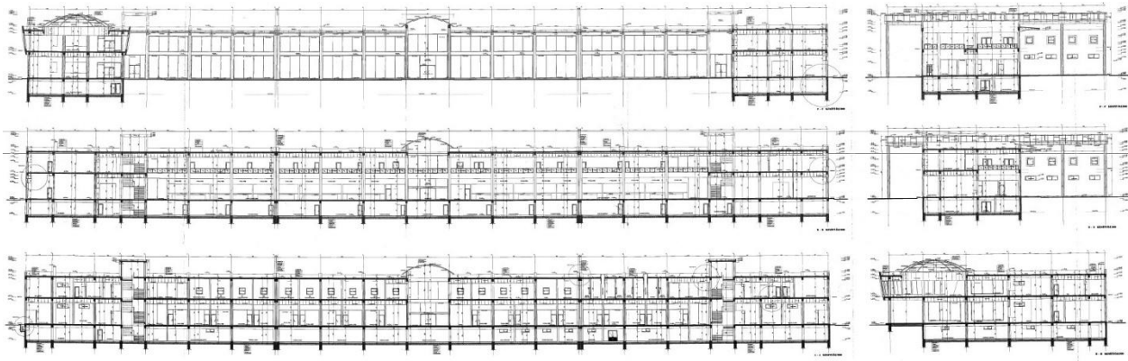
KESİT
