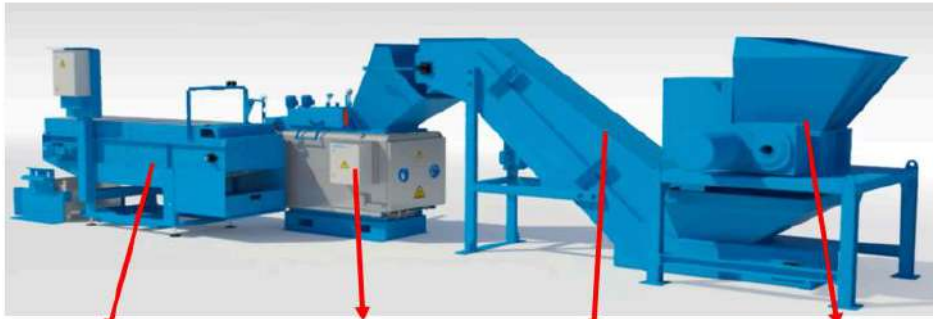
5. Külçe Konveyörü 4. Ergitme Fırını 3. Yolluk Konveyörü 2. Yolluk Kırma Mak.
